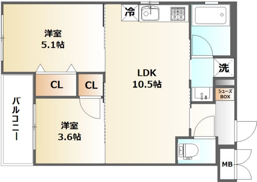
【間取り図】
